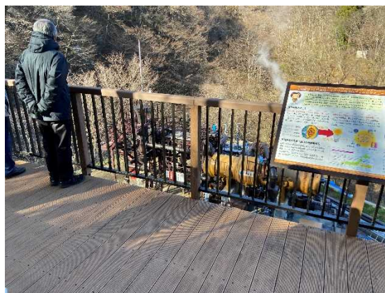
Ptcl.56 バイナリー発電所と説明板
