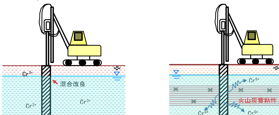
図-1 六価クロムの溶出概念図（左：通常地盤、右：溶出が起る地盤の例）
