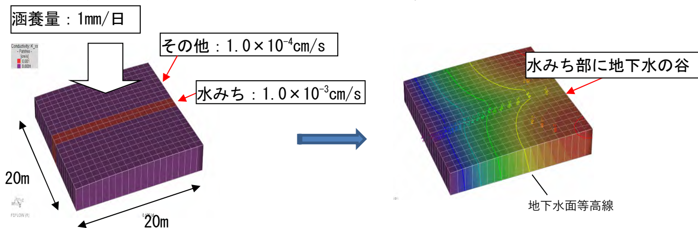
図-1 単純な水みちモデル
