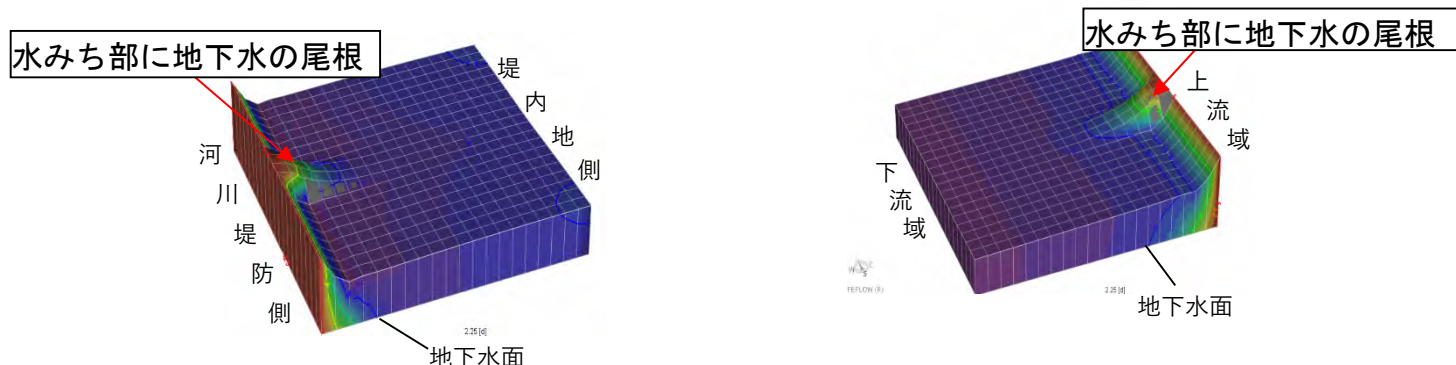
図-3 洪水時の河川堤防沿いの水みち
